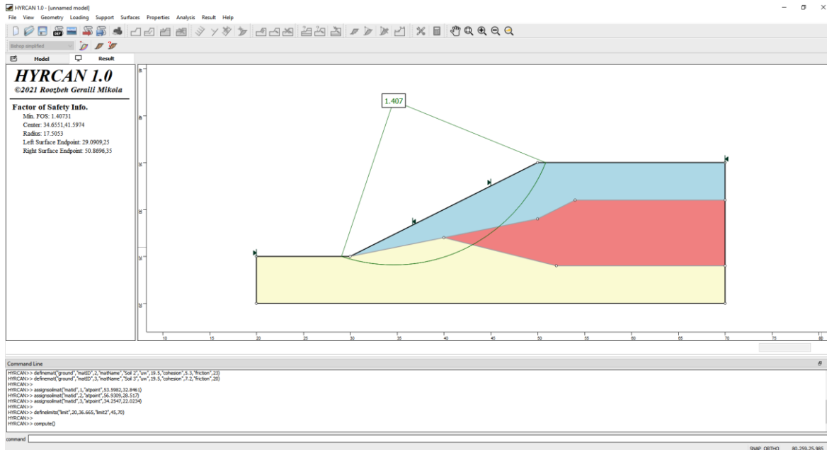
Рисунок 5- Результат автоматического поиска поверхностей скольжения.
