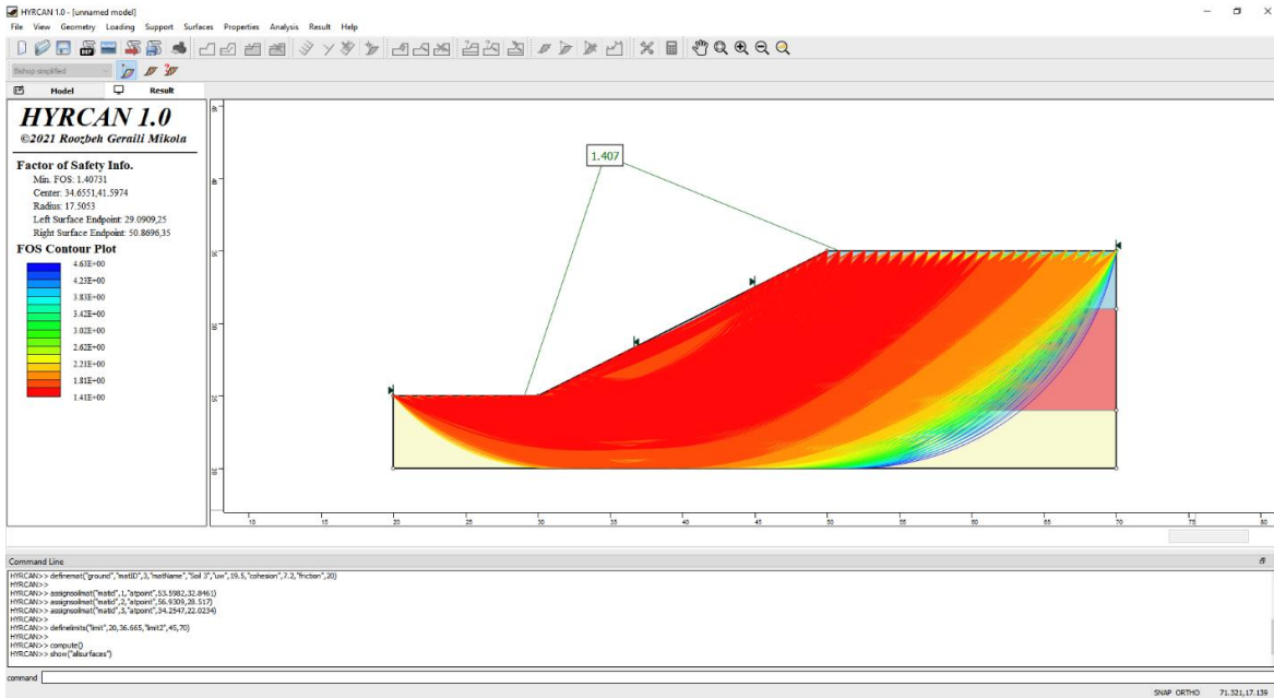
Рисунок 6- Найденные круглоцилиндрические поверхности скольжения – показаны все поверхности.
